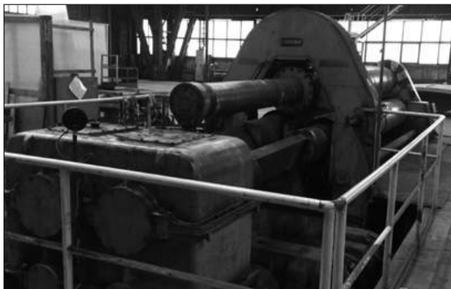
Walcarka z Oddziału Prefabrykatów w hali III wsadowej WBG przed wdrożeniem systemu TPM i po oczyszczeniu zgodnie z przyjętymi zasadami.
